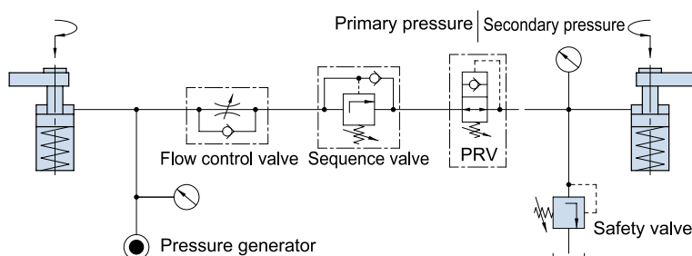
迴路圖 Circuit diagram
