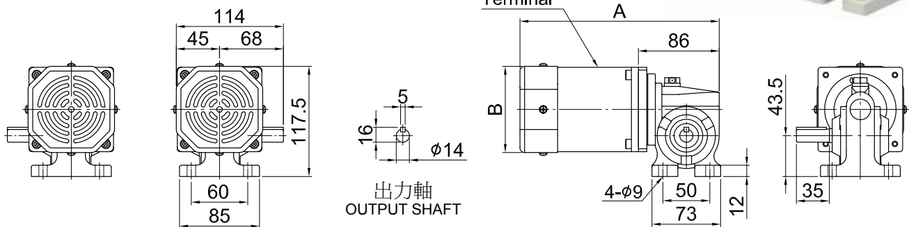
出力軸左方圖 LEFT SHAFT
