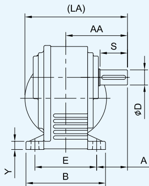
左軸 LEFT SHAFT
