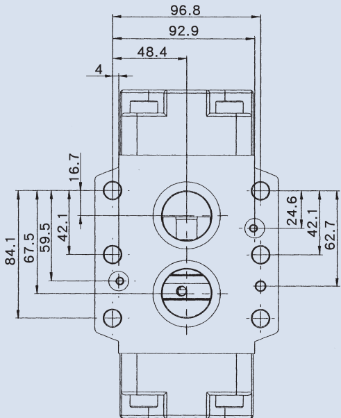
RGM-10, RCGM-10, HGM-10, HCGM-10, CPDGM-10
